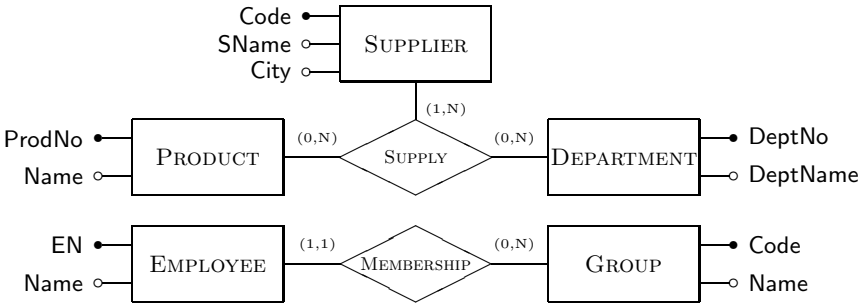
Fig. 2. Two simple ER schemas
